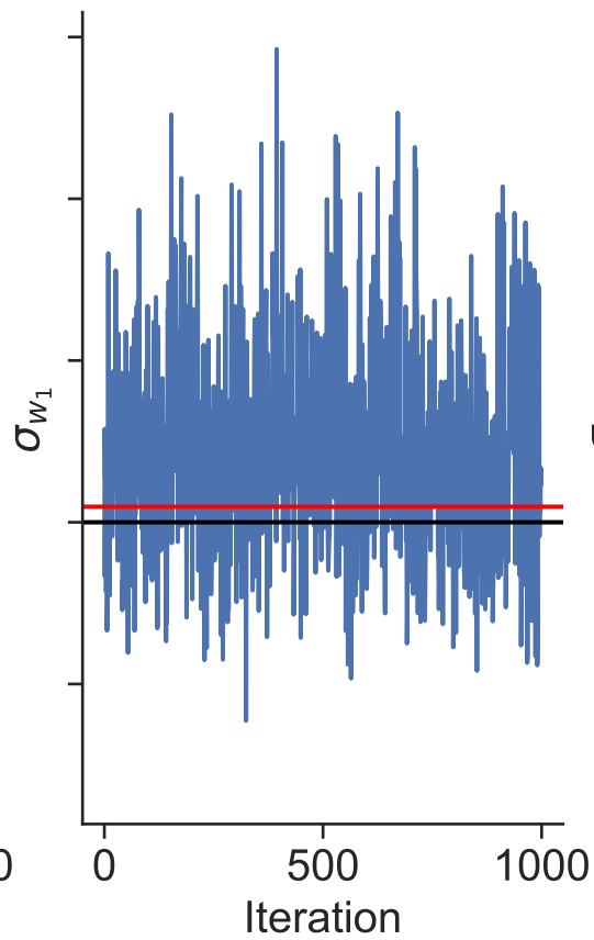
Posterior distributions Dataset 44
