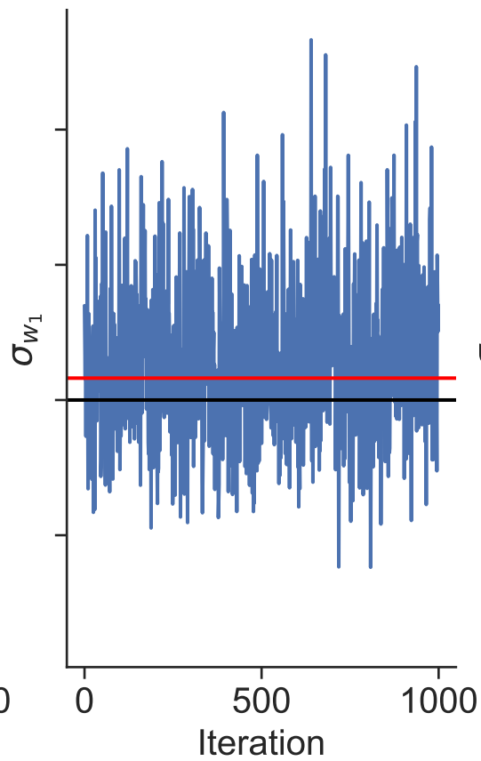
Posterior distributions Dataset 40
